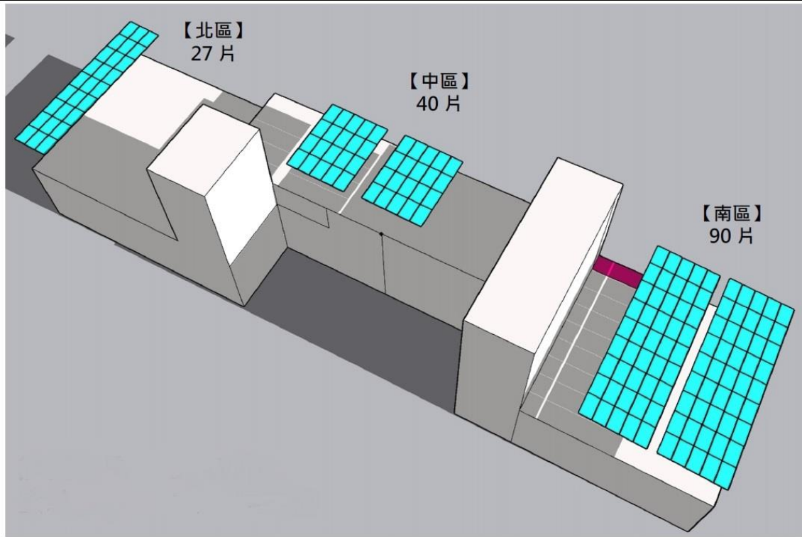
太陽光電發電系統(建置示意圖)
